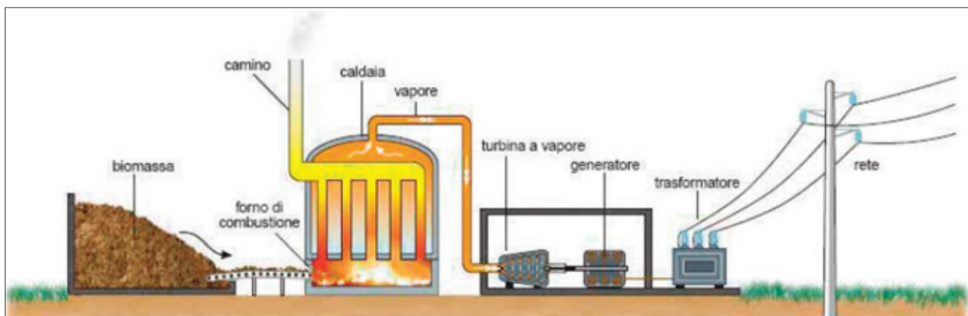
Schema di impianto per la trasformazione di biomasse in energia elettrica.
